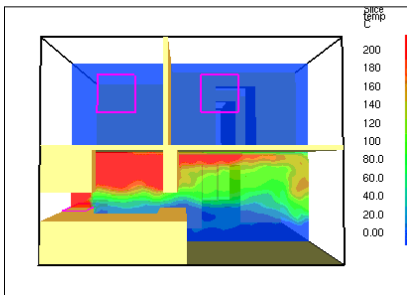
Rysunek 4. Ekran przedstawiający przemieszczanie się warstwy dymu w budynku dwukondygnacyjnym wraz z rozkładem temperatur gorących gazów pożarowych. Symulacja wykonana za pomocą programu Fire Dynamics Simulator i Smokeview.
